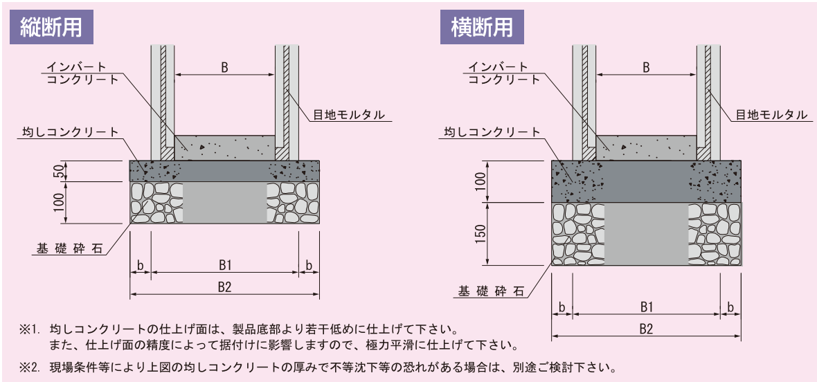
寸法表(縦断用：リボン自由勾配側溝) (10m当り)
