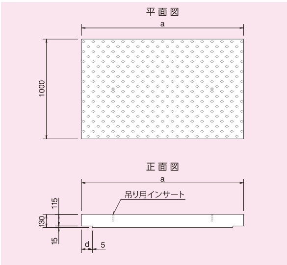
Hi-P水路 床版寸法表
