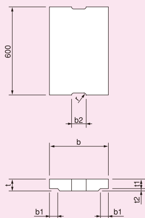
コンクリート蓋 (JIS推奨仕様)
