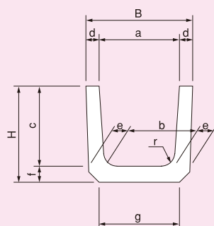
本体 (JIS推奨仕様)
