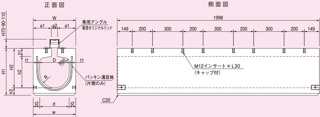
寸法表
