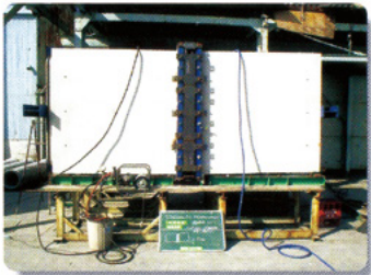
実験状況（曲げ角度1.0°）
