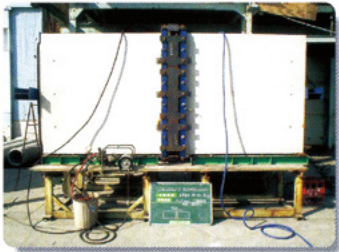
実験状況（抜け出し35mm）
