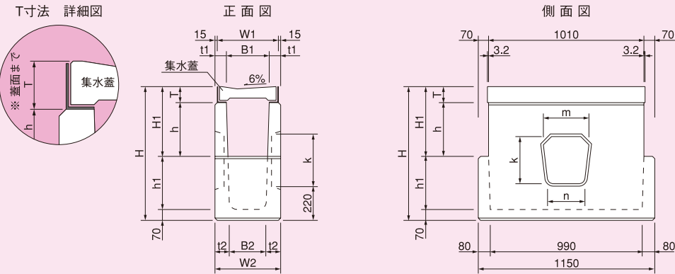
寸法表
