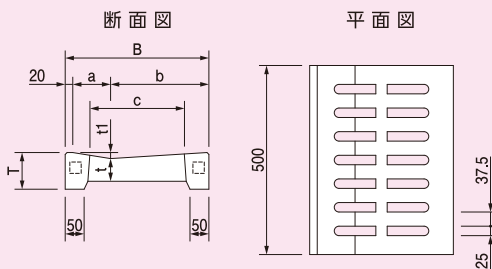
寸法表
