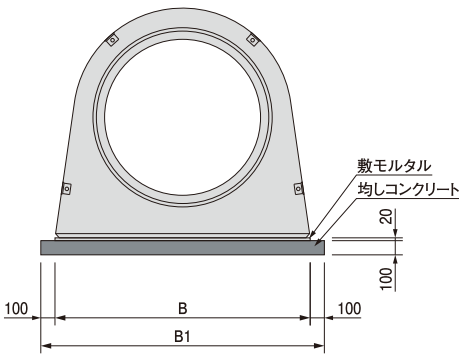
プレキャスト底樋管(本體工) (10m当り)
