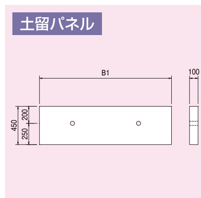
寸法表(土留パネル)
