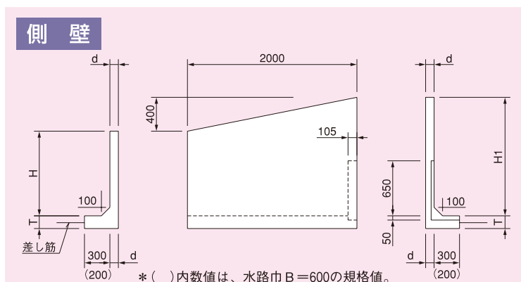
寸法表(側壁)
