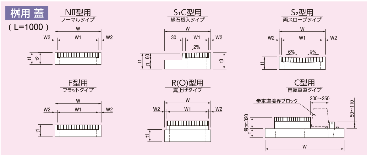
寸法表(柵用 蓋)
