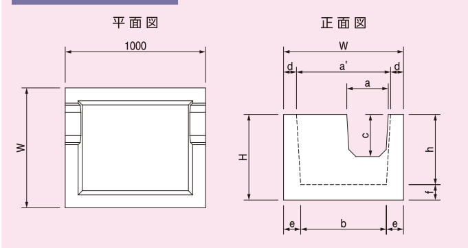
C型専用柵本体
