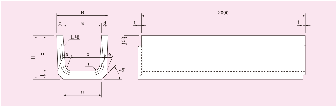
寸法表
