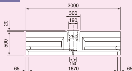
正面図・背面図
