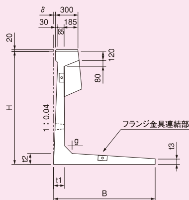
断面図
