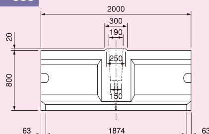
正面図・背面図
