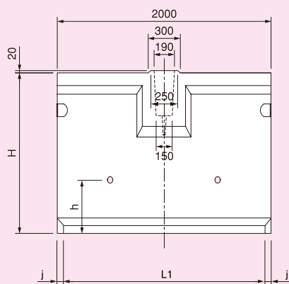
正面図・背面図
