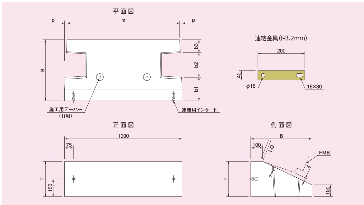
寸法表(3分・4分・5分 共通)
