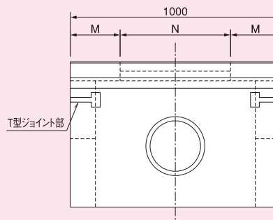
側面図
