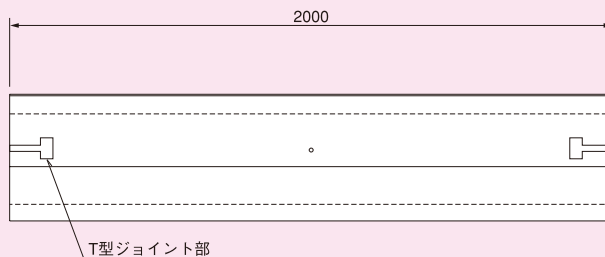
側面図
