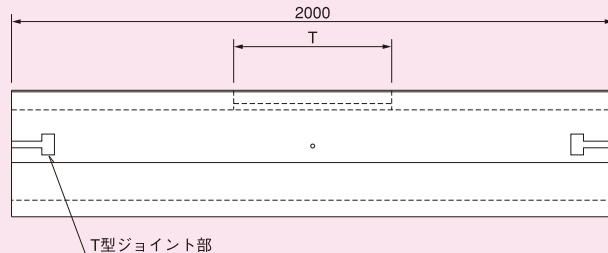
側面図
