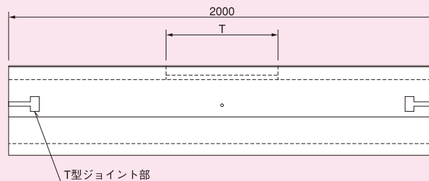
側面図
